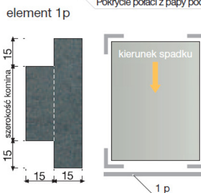
Pokrycie połaci z papy podkładowej
