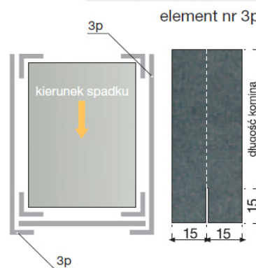
Pokrycie połaci z papy podkładowej
